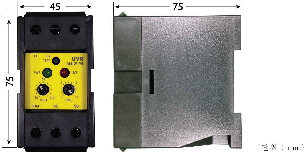
그림1. UVR 외형 및 크기
