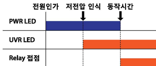
그림2. 동작 CHART
